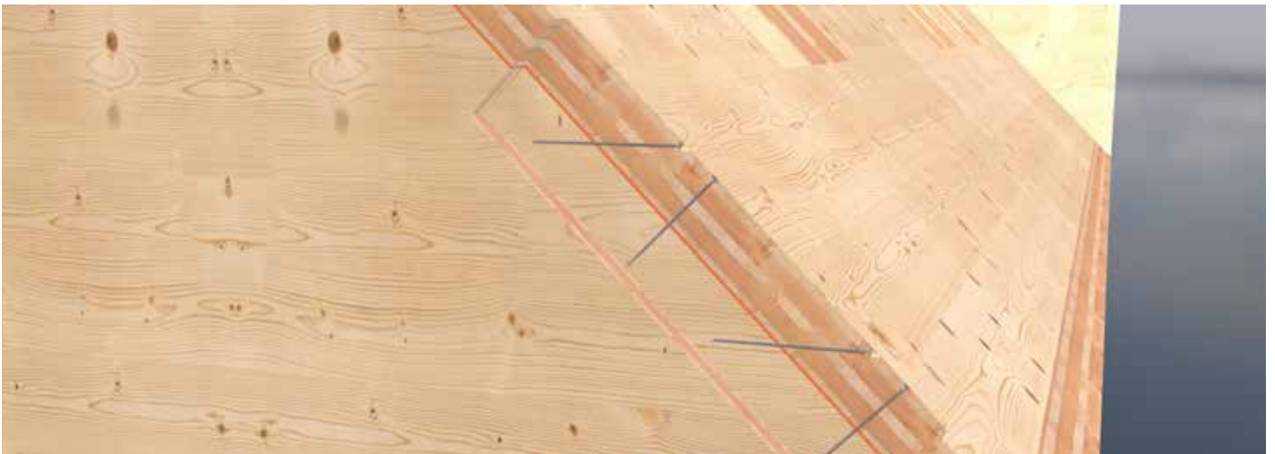
Collegamento del tetto con l'elemento a parete
