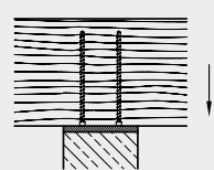
Rinforzo dell'appoggio
