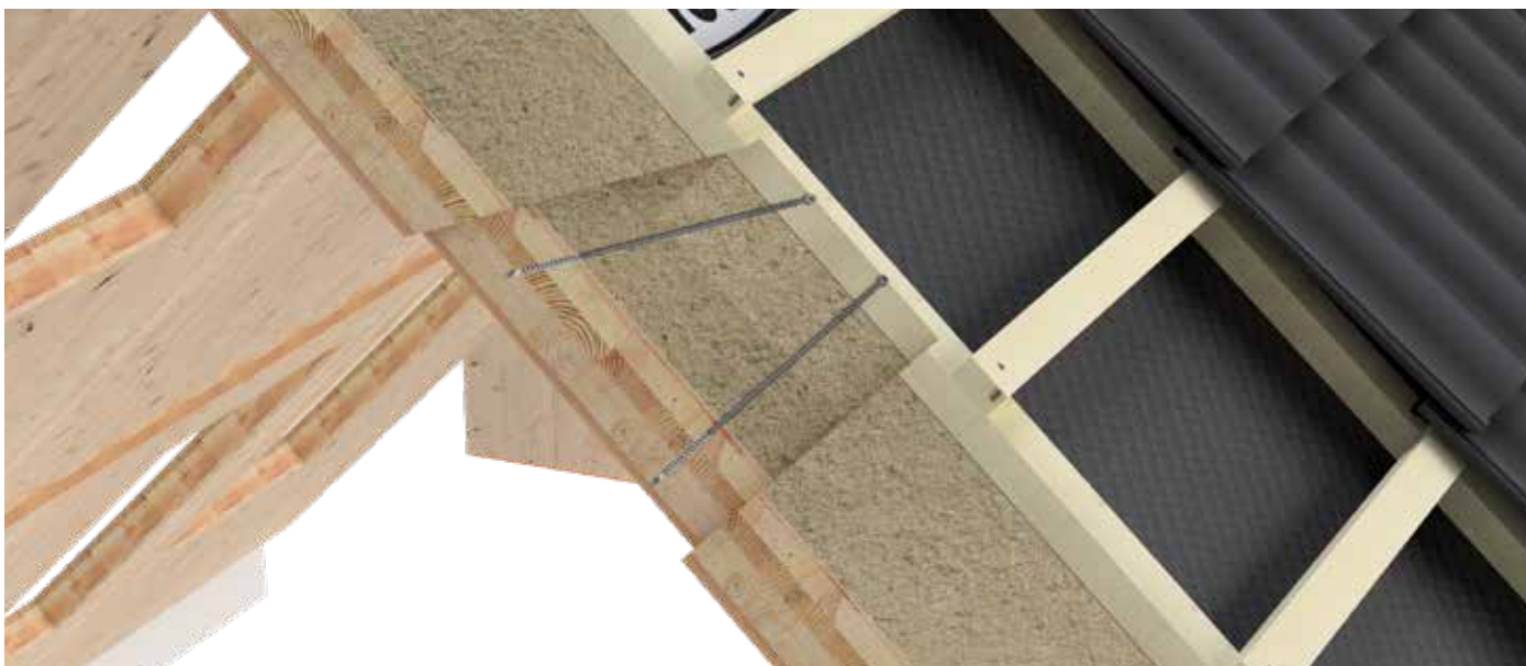
Topduo testa cilindrica per il fissaggio di materiali isolanti
