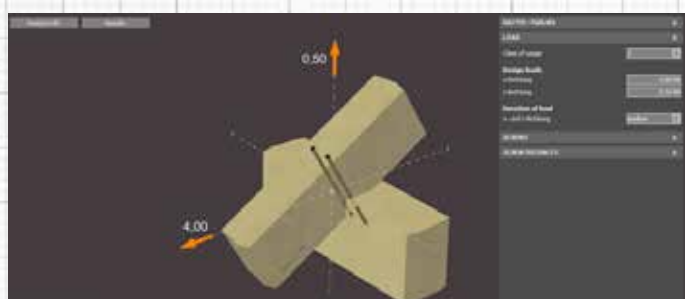
Modulo per il collegamento di travetto inclinato e arcareccio con Paneltwistec e KonstruX
