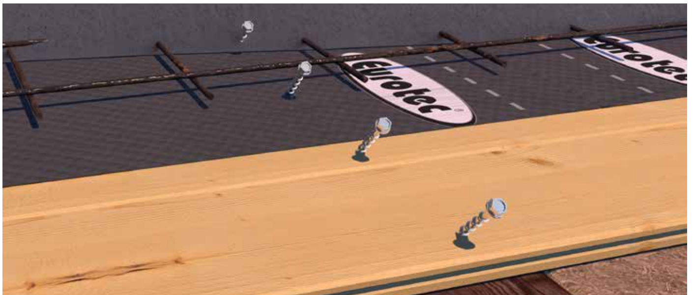
Disaccoppiamento dal rumore dei passi e massetto sul soffitto HBV
