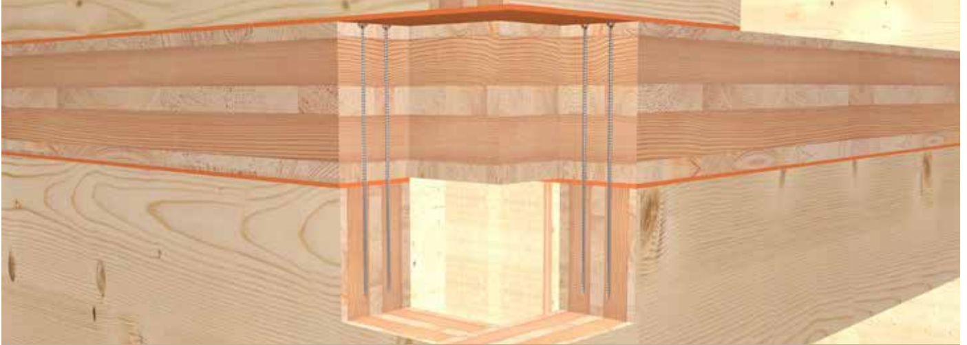
Collegamento dell'elemento a parete con l'elemento di copertura
