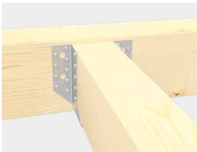
Verbindung zweier Holzbalken mithilfe des Balkenschuhs außen.
