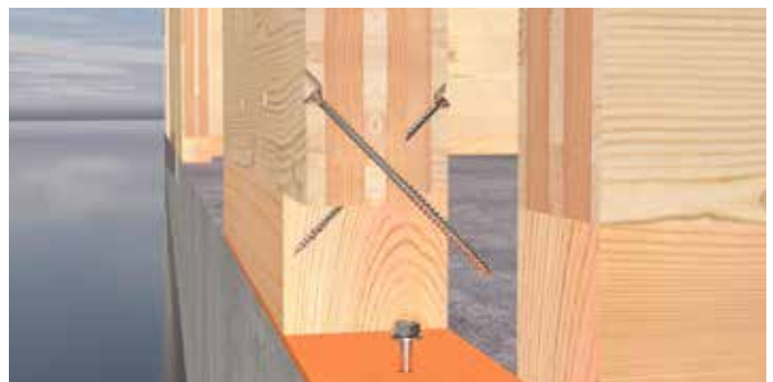
KonstruX zur Verbindung von Wand und Schwellenholz.
