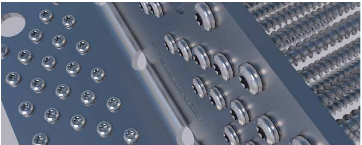
Winkelbeschlagschraube in Systemwinkel CLT.
