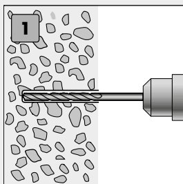
1 Bohrloch erstellen. (Hammerbohren)
