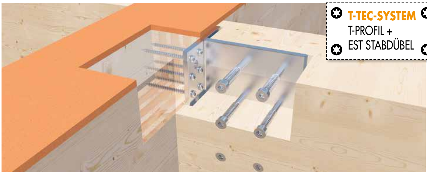
T-Profil in Kombination mit dem EST Stabdübel zur Montage eines Balkens an einer Wand.
