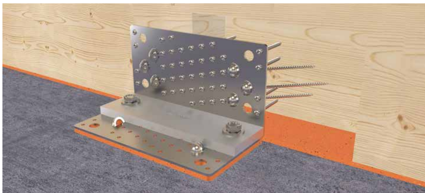
Scherwinkel zur Befestigung einer Wand am Betonfundament.
