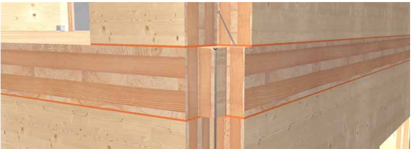
Verbindung von Wand und Holzboden im OG.
