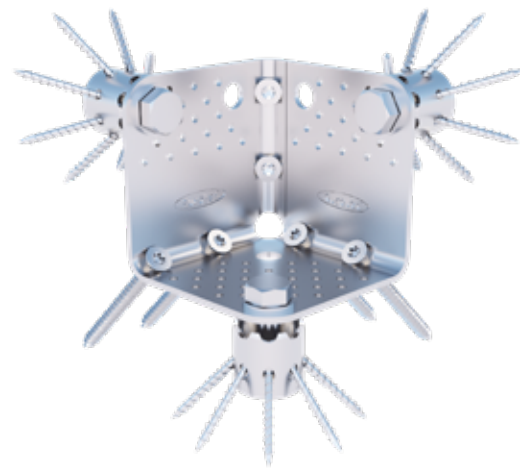
Systeminnenecke CLT mit IdeeFix
