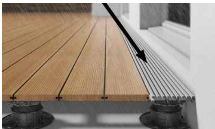
Mit DrainTec wird der Regen kontrolliert abgeleitet und das Regenwasser fließt direkt in den Untergrund.
