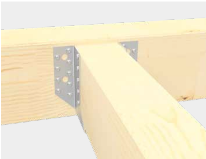
Verbindung zweier Holzbalken mithilfe des Balkenschuhs außen.
