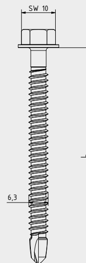
Vista laterale
