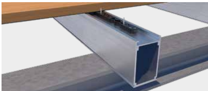
Zamocowanie niewidoczne przez ślizgacz tarasu
