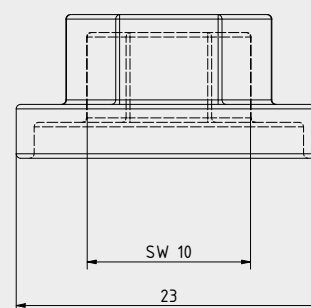
Vista lateral
