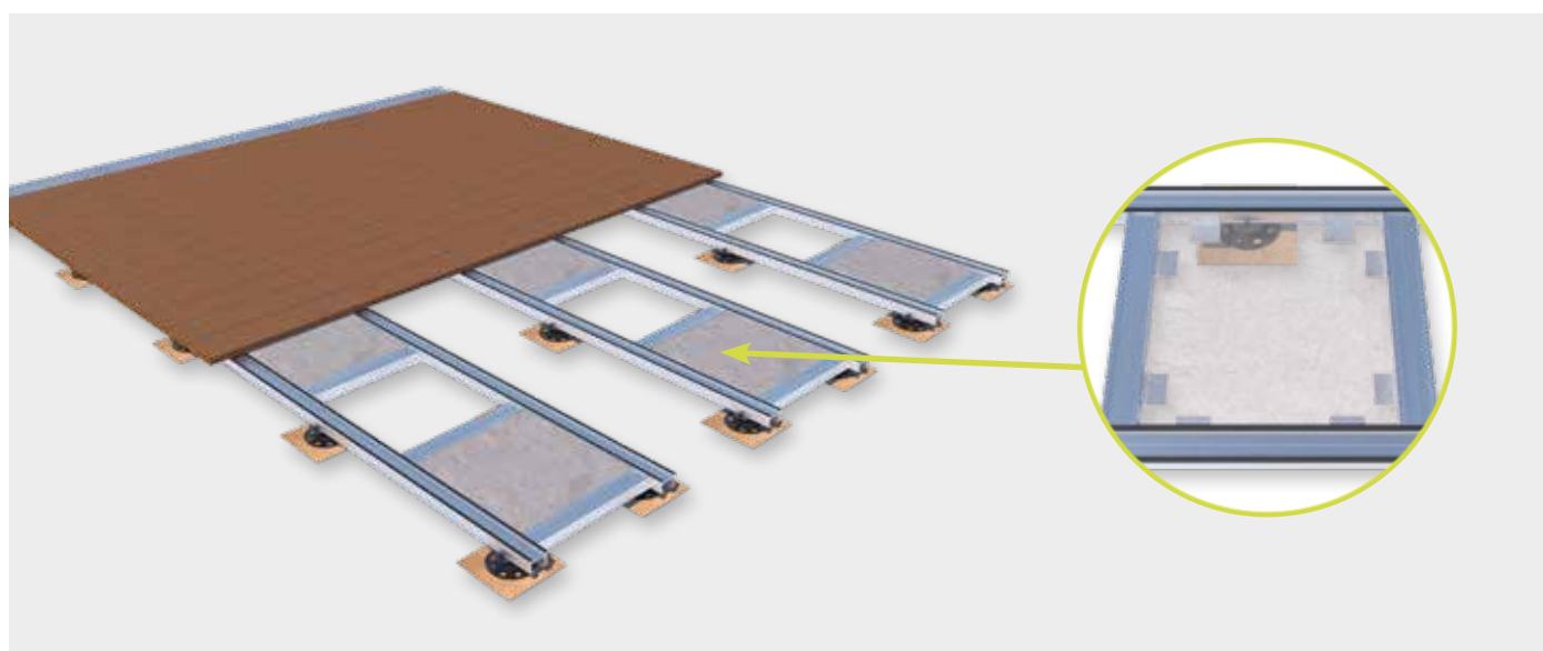
Sujeción contra la succión del viento en terrazas de madera con el uso de losetas apoyadas en las escuadra de sobrecarga
