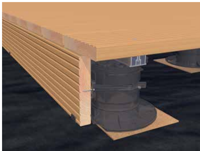
Terminación muy estética gracias al Soporte lateral para terrazas.
