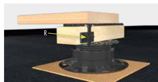
Fijando una tabla de madera a una subestructura de madera utilizando el Conector a presión (R).
