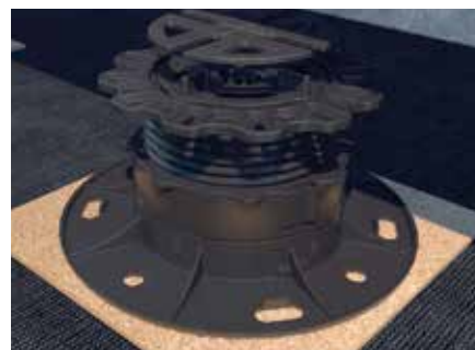
Plot regulable PRO con disco de amortiguación
