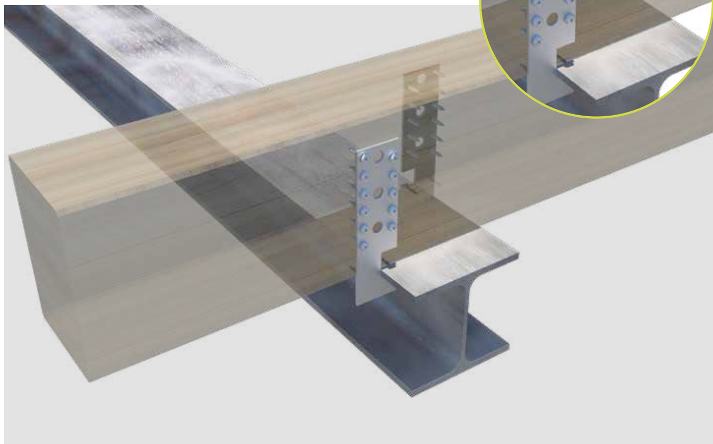
Anclaje para perfiles T usado en una viga laminada doble T.
