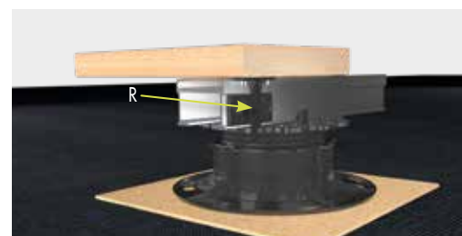
Fijando una tabla de madera al sistema de perfilera de aluminio EVO utilizando el Conector a presión (R).
