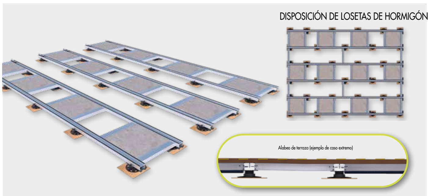
Fijación contra el alabeo causado por condiciones ambientales.
