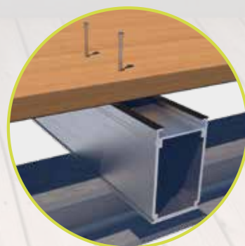
Fijación a vista utilizando tornillo autoperforante para perfiles
