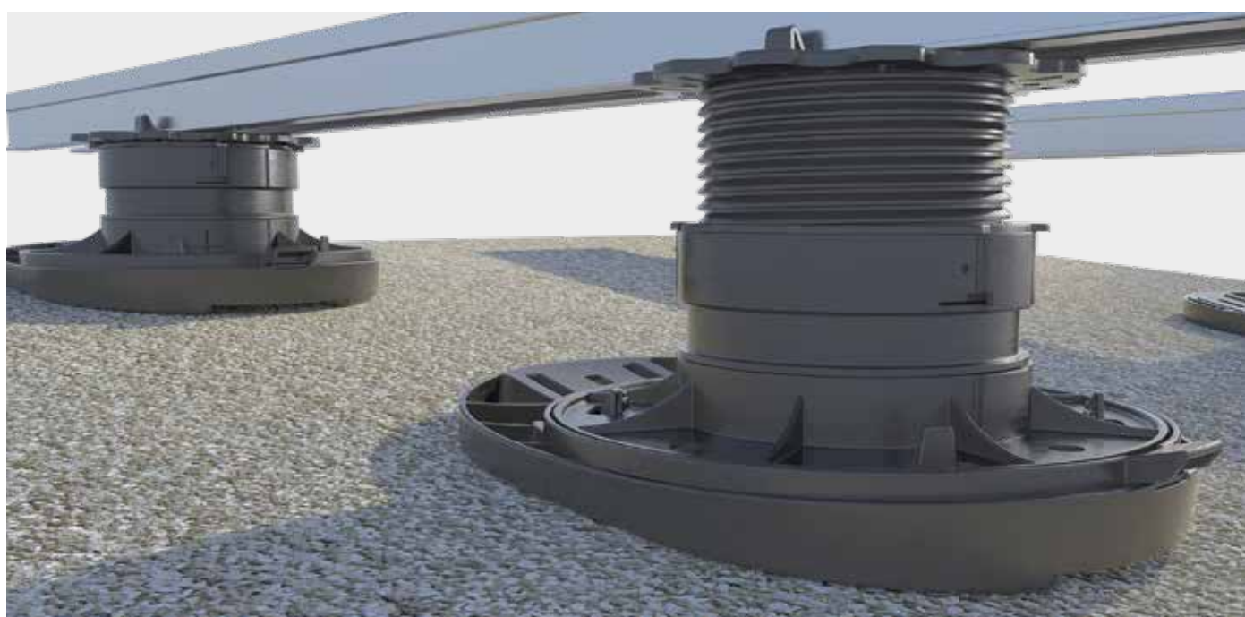
Nivelación de pendientes con el Nivello 2.0
