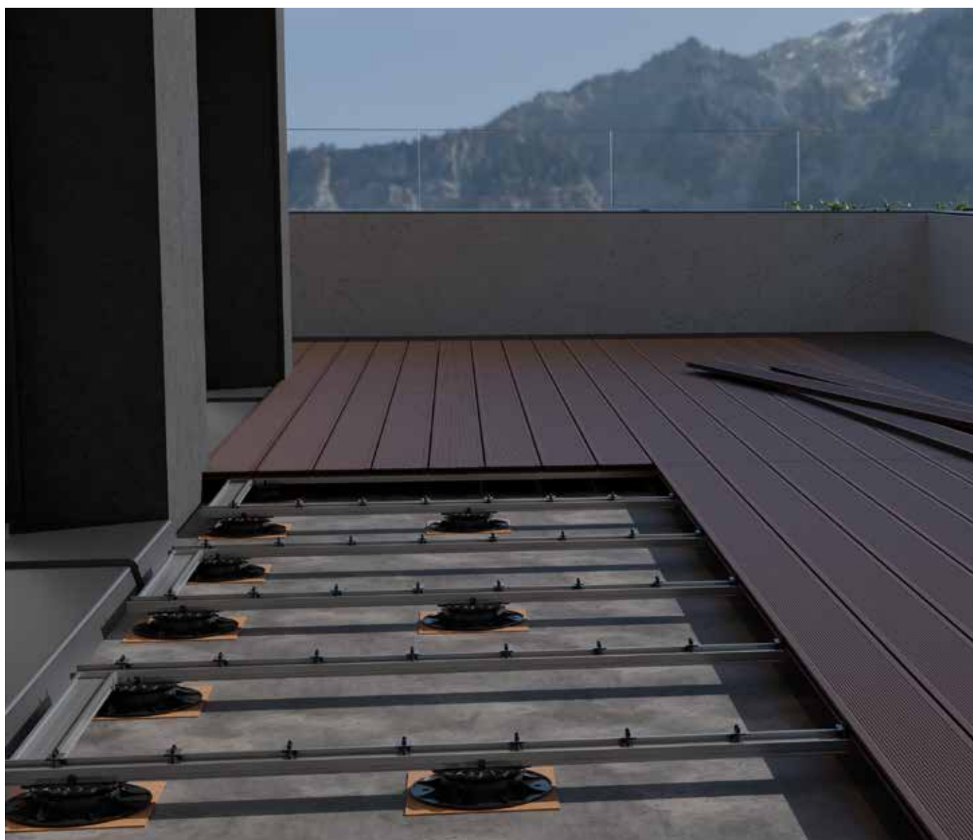
Subestructura con plots regulable PRO, adaptador click 60, sistema de perfilaría de aluminio EVO y grapa Twin
