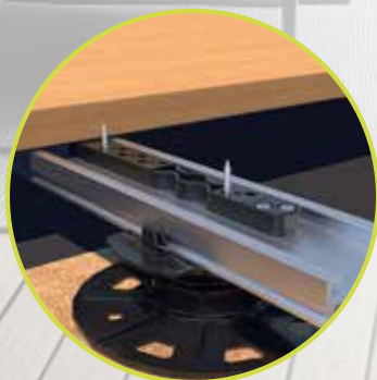
Fijación oculta utilizando juntas deslizantes para terrazas
