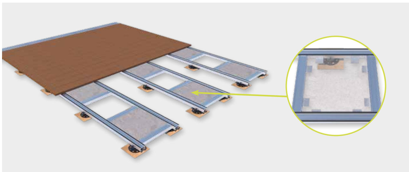
Fijación de terrazas contra la succión del viento, con losetas de hormigón y escuadras de fijación.
