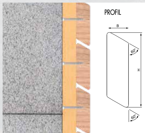
Conexión a la pared con el tornillo para fachadas ZK
