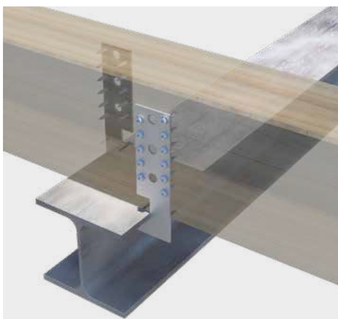
T-Träger Anker in Verbindung mit einem T-Träger.
