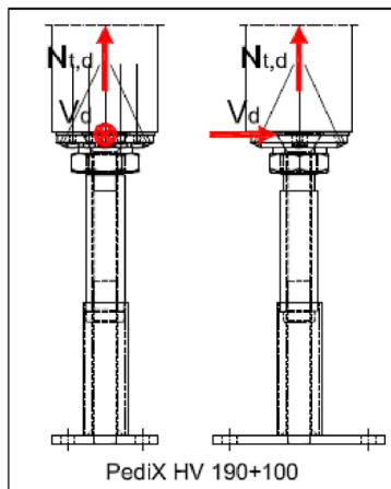
Abbildung B-3: Tragfähigkeiten des Stützenfußes PediX HV 190+100 bei Interaktion von Zug- und Querkraftbeanspruchungen für angenommene Teilsicherheitsbeiwerte \gamma_M=1,3 , \gamma_{M0}=1,0 , \gamma_{M1}=1,1 und \gamma_{M2}=1,25
