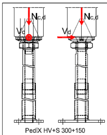
Abbildung B-10: Tragfähigkeiten des Stützenfußes PediX HV+S 300+150 bei Interaktion von Druck- und Querkraftbeanspruchungen für angenommene Teilsicherheitsbeiwerte \gamma_M=1,3 , \gamma_{M0}=1,0 , \gamma_{M1}=1,1 und \gamma_{M2}=1,25
