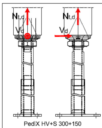
Abbildung B-9: Tragfähigkeiten des Stützenfußes PediX HV+S 300+150 bei Interaktion von Zug- und Querkraftbeanspruchungen für angenommene Teilsicherheitsbeiwerte \gamma_M=1,3 , \gamma_{M0}=1,0 , \gamma_{M1}=1,1 und \gamma_{M2}=1,25
