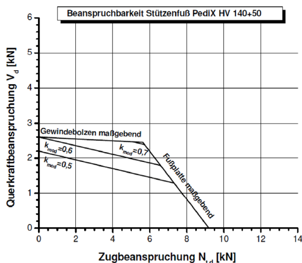
Abbildung B-1: Tragfähigkeiten des Stützenfußes PediX HV 140+50 bei Interaktion von Zug- und Querkraftbeanspruchungen für angenommene Teilsicherheitsbeiwerte \gamma_M=1,3 , \gamma_{M0}=1,0 , \gamma_{M1}=1,1 und \gamma_{M2}=1,25
