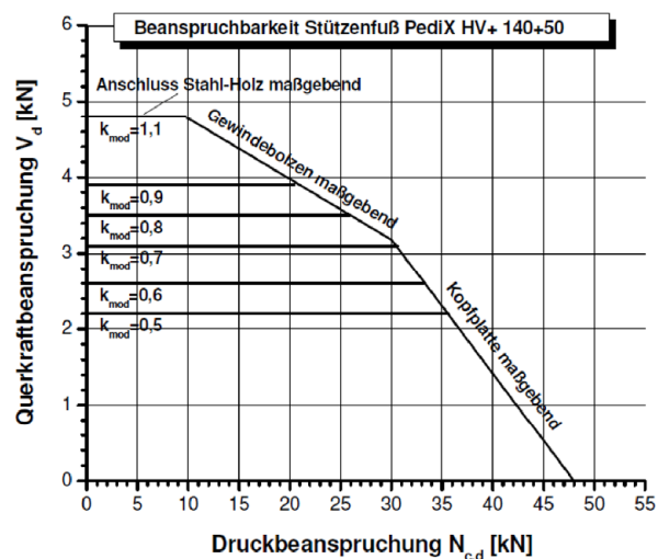
Abbildung B-6: Tragfähigkeiten des Stützenfußes PediX HV+ 140+50 bei Interaktion von Druck- und Querkraftbeanspruchungen für angenommene Teilsicherheitsbeiwerte \gamma_M=1,3 , \gamma_{M0}=1,0 , \gamma_{M1}=1,1 und \gamma_{M2}=1,25
