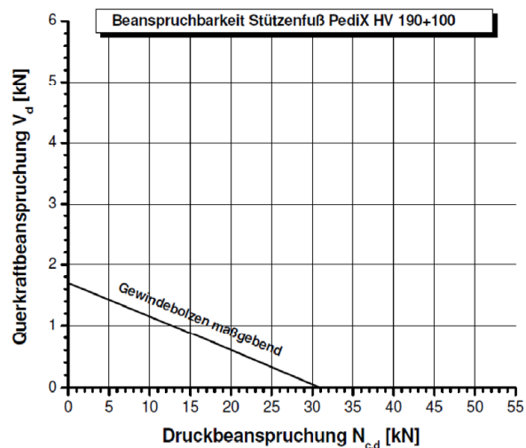
Abbildung B-4: Tragfähigkeiten des Stützenfußes PediX HV 190+100 bei Interaktion von Druck- und Querkraftbeanspruchungen für angenommene Teilsicherheitsbeiwerte \gamma_M=1,3 , \gamma_{M0}=1,0 , \gamma_{M1}=1,1 und \gamma_{M2}=1,25
