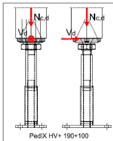
Abbildung B-8: Tragfähigkeiten des Stützenfußes PediX HV+ 190+100 bei Interaktion von Druck- und Querkraftbeanspruchungen für angenommene Teilsicherheitsbeiwerte \gamma_M=1,3 , \gamma_{M0}=1,0 , \gamma_{M1}=1,1 und \gamma_{M2}=1,25
