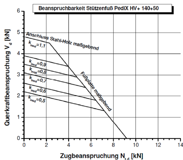
Abbildung B-5: Tragfähigkeiten des Stützenfußes PediX HV+ 140+50 bei Interaktion von Zug- und Querkraftbeanspruchungen für angenommene Teilsicherheitsbeiwerte \gamma_M=1,3 , \gamma_{M0}=1,0 , \gamma_{M1}=1,1 und \gamma_{M2}=1,25
