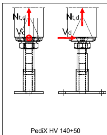
Abbildung B-1: Tragfähigkeiten des Stützenfußes PediX HV 140+50 bei Interaktion von Zug- und Querkraftbeanspruchungen für angenommene Teilsicherheitsbeiwerte \gamma_M=1,3 , \gamma_{M0}=1,0 , \gamma_{M1}=1,1 und \gamma_{M2}=1,25
