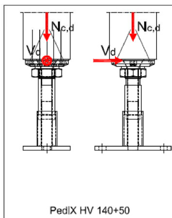
Abbildung B-2: Tragfähigkeiten des Stützenfußes PediX HV 140+50 bei Interaktion von Druck- und Querkraftbeanspruchungen für angenommene Teilsicherheitsbeiwerte \gamma_M=1,3 , \gamma_{M0}=1,0 , \gamma_{M1}=1,1 und \gamma_{M2}=1,25
