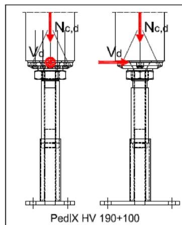
Abbildung B-4: Tragfähigkeiten des Stützenfußes PediX HV 190+100 bei Interaktion von Druck- und Querkraftbeanspruchungen für angenommene Teilsicherheitsbeiwerte \gamma_M=1,3 , \gamma_{M0}=1,0 , \gamma_{M1}=1,1 und \gamma_{M2}=1,25
