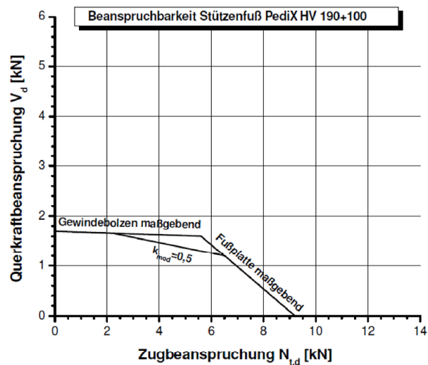
Abbildung B-3: Tragfähigkeiten des Stützenfußes PediX HV 190+100 bei Interaktion von Zug- und Querkraftbeanspruchungen für angenommene Teilsicherheitsbeiwerte \gamma_M=1,3 , \gamma_{M0}=1,0 , \gamma_{M1}=1,1 und \gamma_{M2}=1,25
