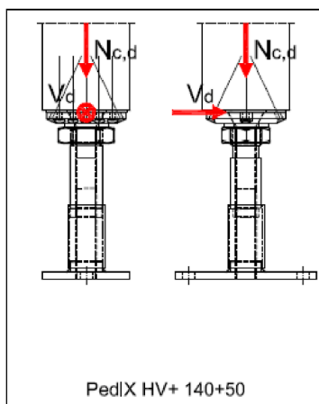
Abbildung B-6: Tragfähigkeiten des Stützenfußes PediX HV+ 140+50 bei Interaktion von Druck- und Querkraftbeanspruchungen für angenommene Teilsicherheitsbeiwerte \gamma_M=1,3 , \gamma_{M0}=1,0 , \gamma_{M1}=1,1 und \gamma_{M2}=1,25
