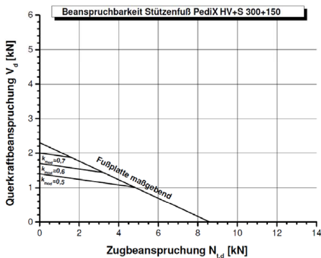
Abbildung B-9: Tragfähigkeiten des Stützenfußes PediX HV+S 300+150 bei Interaktion von Zug- und Querkraftbeanspruchungen für angenommene Teilsicherheitsbeiwerte \gamma_M=1,3 , \gamma_{M0}=1,0 , \gamma_{M1}=1,1 und \gamma_{M2}=1,25
