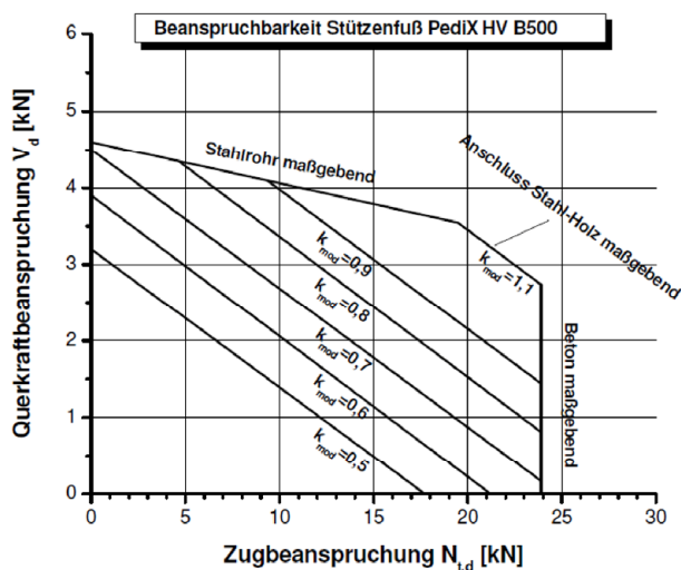
Abbildung B-11: Tragfähigkeiten des Stützenfußes PediX HV B500 bei Interaktion von Zug- und Querkraftbeanspruchungen für angenommene Teilsicherheitsbeiwerte \gamma_M = 1,3 , \gamma_{M0} = 1,0 , \gamma_{M1} = 1,1 und \gamma_C = 1,50
