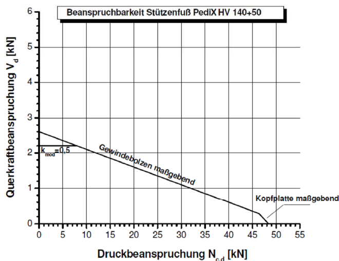
Abbildung B-2: Tragfähigkeiten des Stützenfußes PediX HV 140+50 bei Interaktion von Druck- und Querkraftbeanspruchungen für angenommene Teilsicherheitsbeiwerte \gamma_M=1,3 , \gamma_{M0}=1,0 , \gamma_{M1}=1,1 und \gamma_{M2}=1,25
