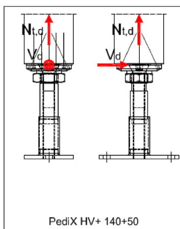
Abbildung B-5: Tragfähigkeiten des Stützenfußes PediX HV+ 140+50 bei Interaktion von Zug- und Querkraftbeanspruchungen für angenommene Teilsicherheitsbeiwerte \gamma_M=1,3 , \gamma_{M0}=1,0 , \gamma_{M1}=1,1 und \gamma_{M2}=1,25
