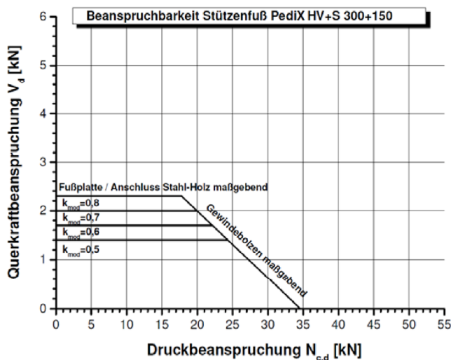
Abbildung B-10: Tragfähigkeiten des Stützenfußes PediX HV+S 300+150 bei Interaktion von Druck- und Querkraftbeanspruchungen für angenommene Teilsicherheitsbeiwerte \gamma_M=1,3 , \gamma_{M0}=1,0 , \gamma_{M1}=1,1 und \gamma_{M2}=1,25
