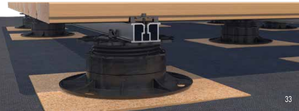
M-Clip
