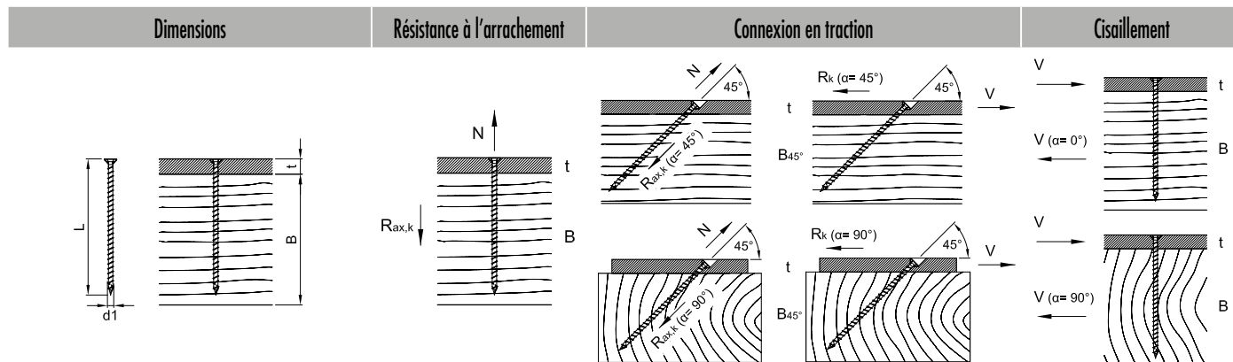
Valeur caractéristique de la capacité de charge de l'assemblage R_{ax,k} selon ETA-11/0024
