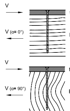
Valeur caractéristique de la capacité de charge de l'assemblage R_k selon ETA-11/0024
