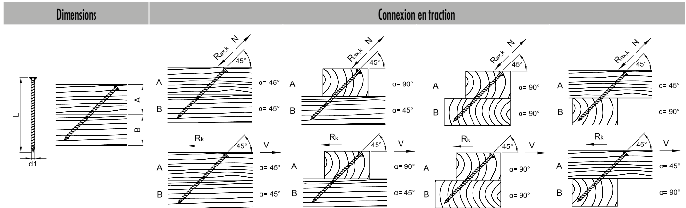
Valeur caractéristique de la capacité de charge de l'assemblage R_{ax,k} et/ou R_k selon ETA-11/0024
