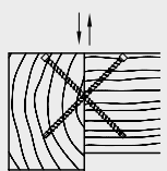
Fixation poutre maîtresse/poutre auxiliaire
