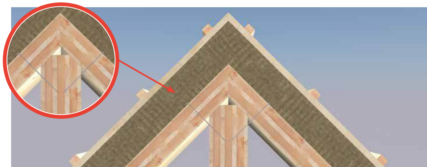
Panneaux de toiture en onglet – Vissage avec la panne faîtière
