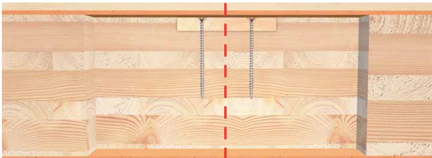
KonstruX pour connexion du mur et du plafond à l'étage
