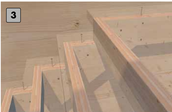
Poser les marches sur la crémaillère.
