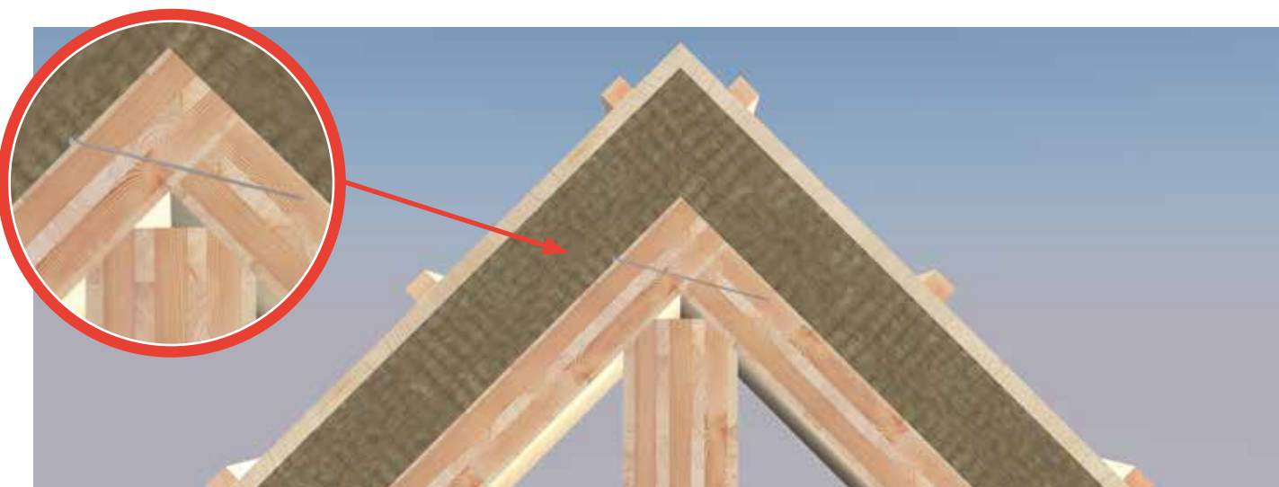
Panneaux de toiture juxtaposés – vissage en biais
