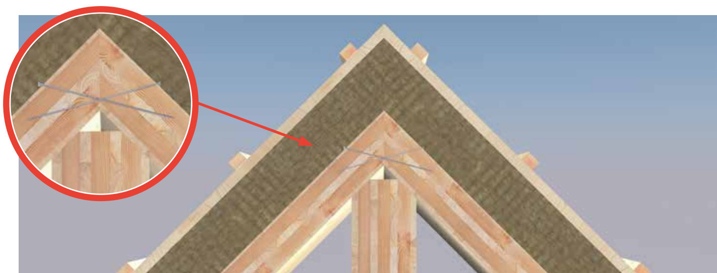
Panneaux de toiture en onglet – vissage en biais
