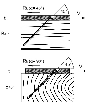
Valeur caractéristique de la capacité de charge de l'assemblage R_{k} et/ou R_k selon ETA-11/0024
