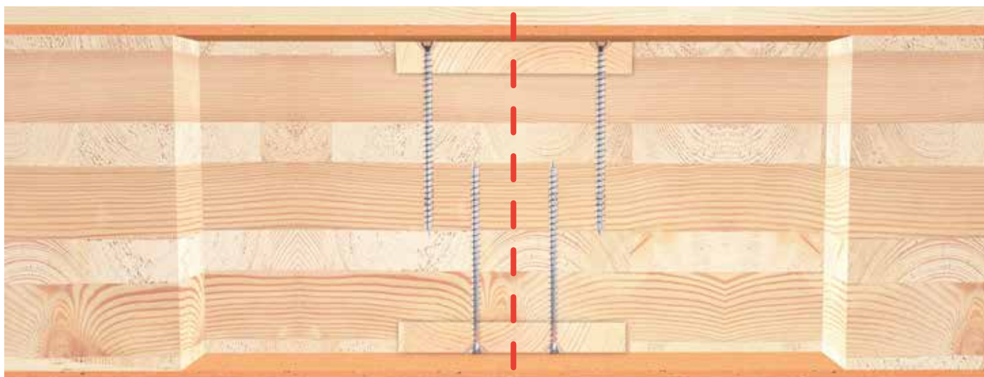
Assemblage d'éléments de plafond moyennant un bois de jointure externe
