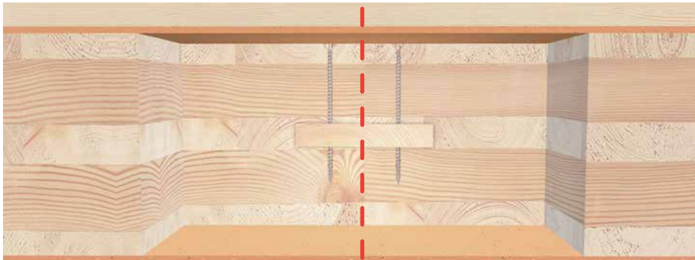
Assemblage d'éléments de plafond moyennant un bois de jointure interne
