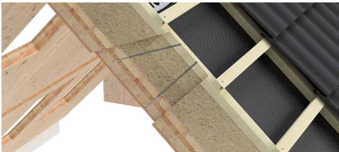
Topduo à tête cylindrique pour la fixation de matériau d'isolation
