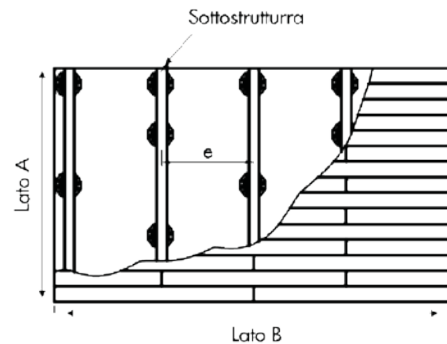
Sottostruttura con profilo in alluminio
