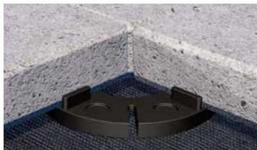
Esempio di applicazione cuscinetto piano EPDM
