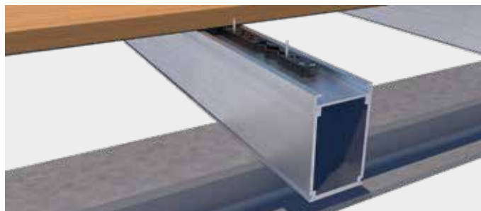
Avvitatura invisibile con elemento scorrevole per terrazze
