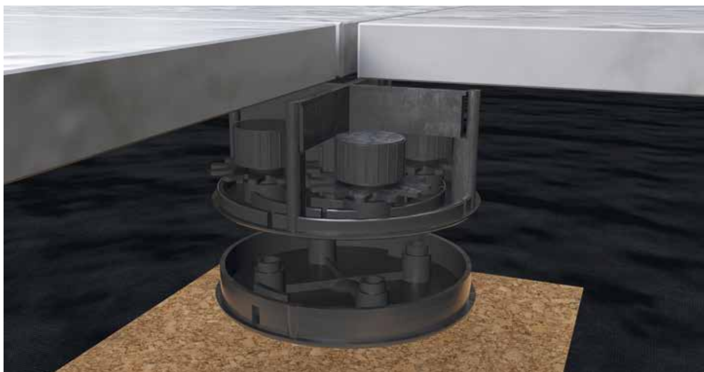
Supporto Quattro con adattatore
