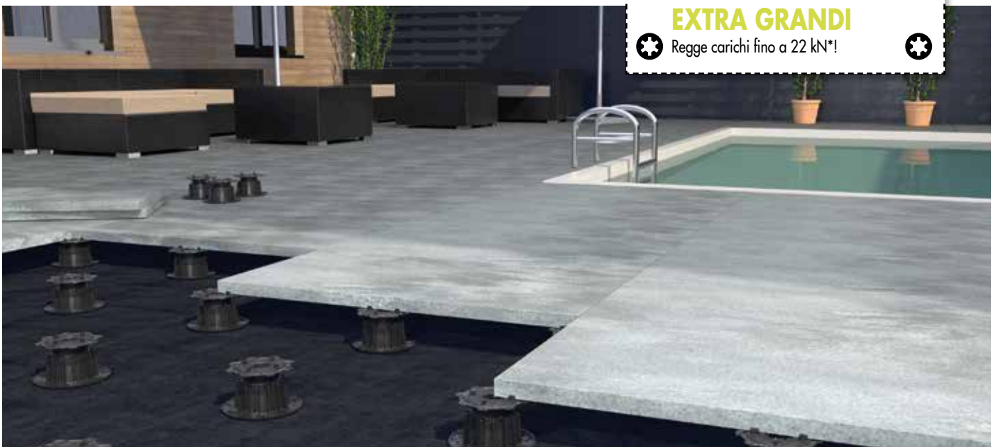
Immagine relativa all'utilizzo terrazza in pietra con piedi regolabili GIANT
