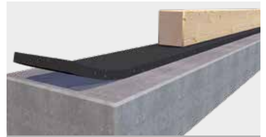
Esempio di applicazione Rolfi rotolo
