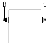
Traglasttabelle für Brettspertholz Wandplatten seitlich an Stirnfläche mit 15 cm Randabstand angeschlagen [min.b x l x d = 50 x 50 x 9]
