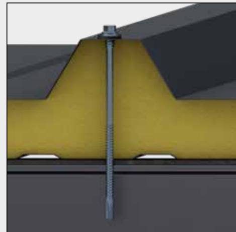
Fixation dans une membrure supérieure sans appareil d'appui sphérique
