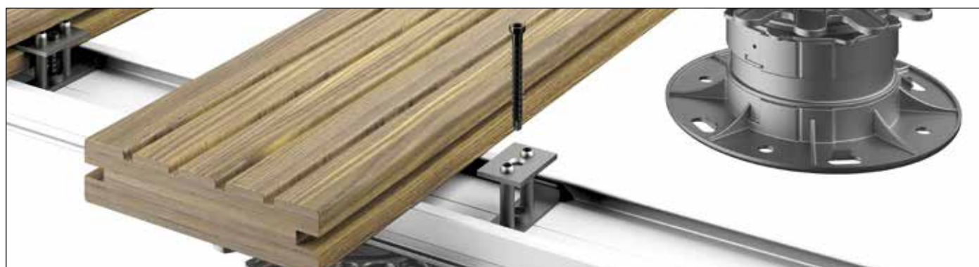
Niewidoczne mocowanie deski drewnianej za pomocą uchwyty systemowego Twin.
