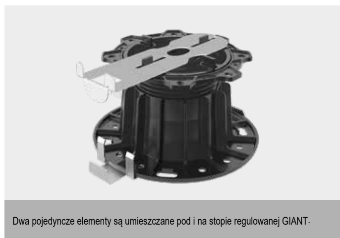
Umieszczanie płyt kamiennych w prowadnicach pojedynczego podparcia wykończenia obrzeży.
