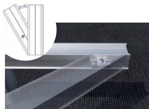
Przykład zastosowania łącznik zabezpieczający położenie EVO
