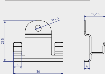
Klips fasadowy Rhombus Starter
