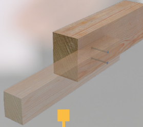
PARALLELANSCHLUSS
