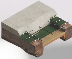
HOLZ-BETON- VERBUND
