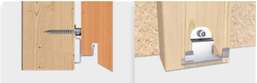
Fassadenclip für Rhombus-Profil Starter Anwendung an vertikaler Holz-Unterkonstruktion
